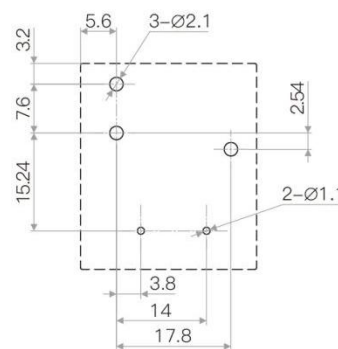
安装孔图(底视图)/Installation hole drawing(Bottom view) 未注公差/Tolerance:±0.1
