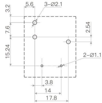
安装孔图(底视图)/Installation hole drawing(Bottom view) 未注公差/Tolerance:±0.1
